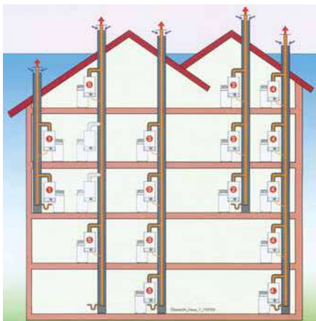
Koncentrični LAS, protustrujni.
