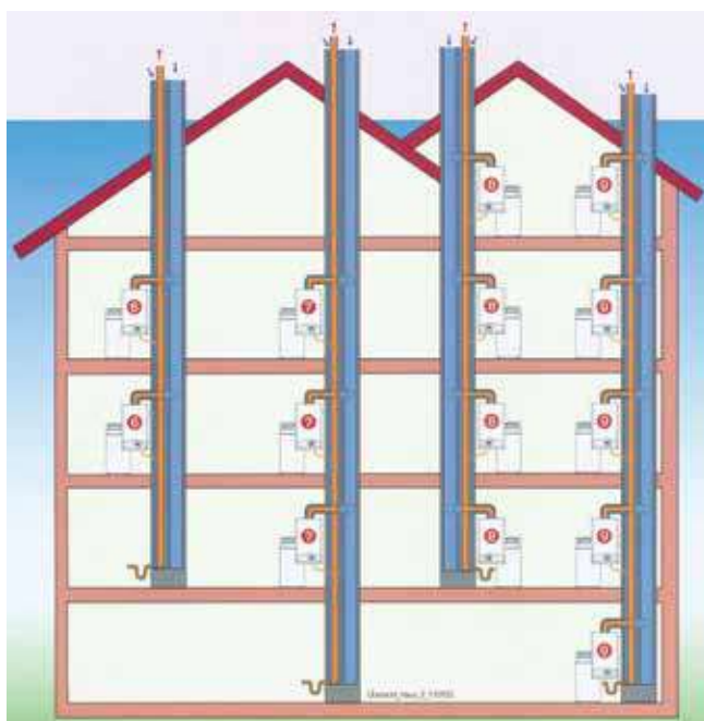
Dvokanalni LAS, paralelni.
